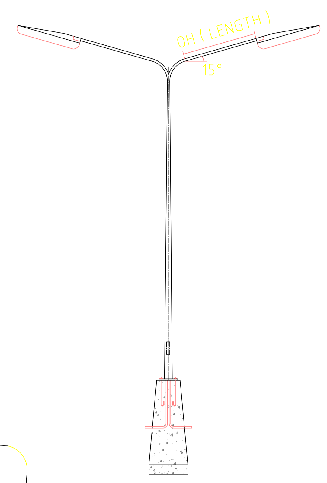
DETALHE - POSTE COM LUMINÁRIAS LED SEM ESCALA
